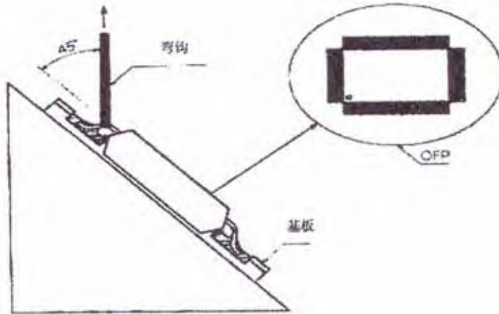
图9 QFP引线焊点45度角拉伸试验示意图
